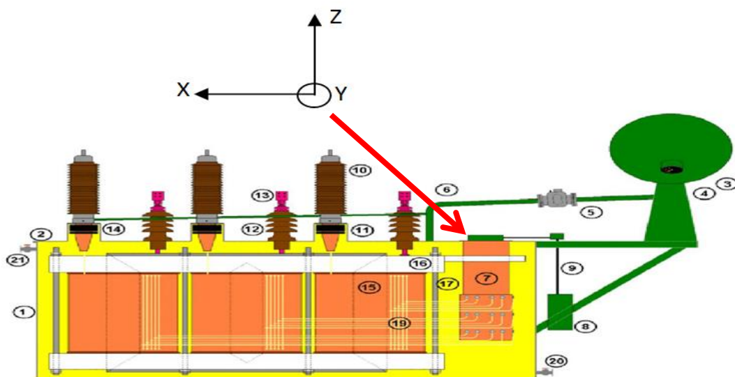
Figure 6: Emplacement du capteur sur la tête du CPEC
