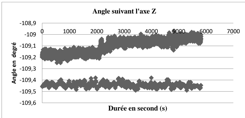
Figure 15: Valeur des angles durant le fonctionnement du transformateur selon l'axe Z
