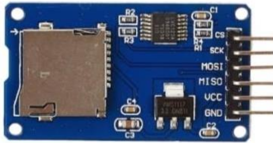
Figure 4: Module micro carte SD
