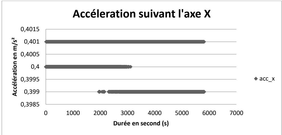
Figure 7: Valeur de l'accélération durant le fonctionnement du transformateur selon l'axe X
