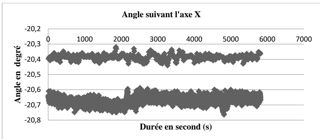
Figure 13: Valeur des angles durant le fonctionnement du transformateur selon l'axe X
